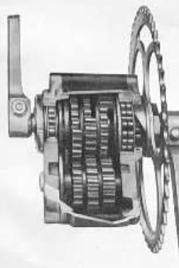
Querschnitt des Modells 1947 Coupe du modèle 1947
