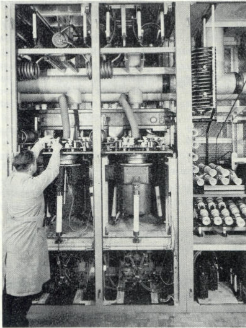
Fig. 2 Teilansicht der HF-Endstufe
