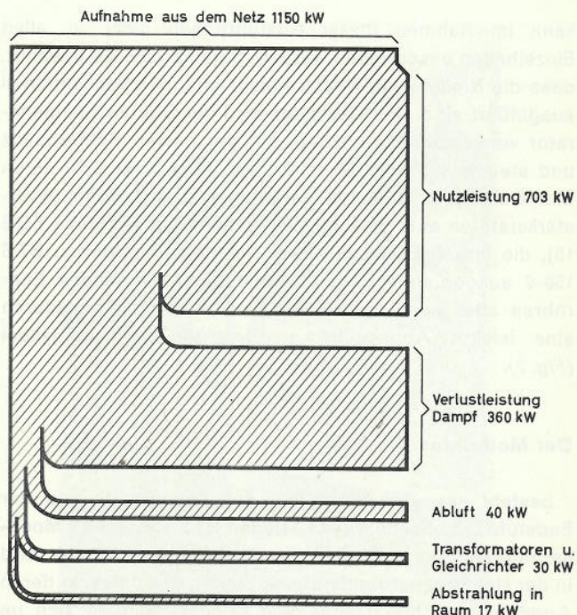
Fig. 1 Leistungsbilanz eines 500-kW-Senders. Modulationsgrad m = 90\%
